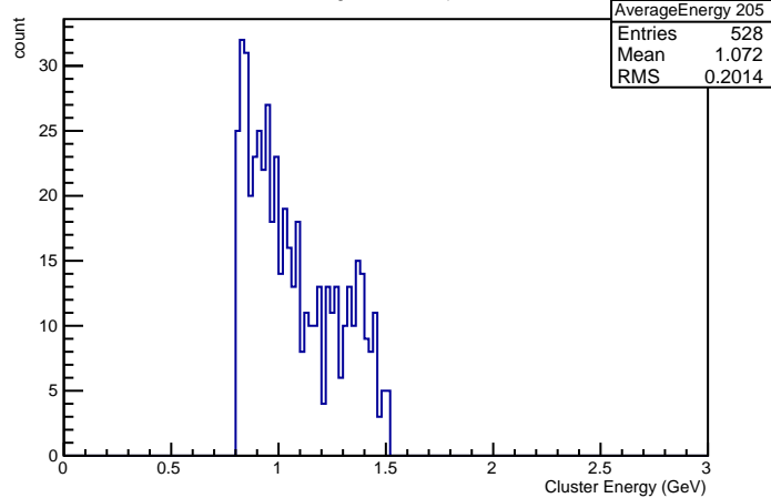
Cluster Energies in Crystal nr 205
