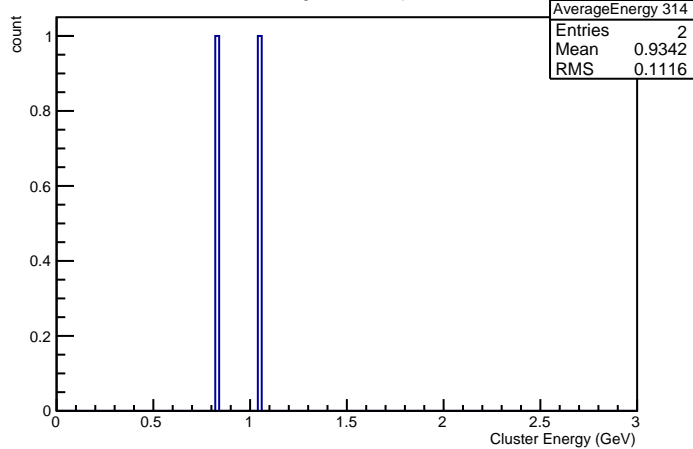
Cluster Energies in Crystal nr 314
