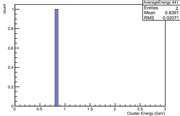
Cluster Energies in Crystal nr 441
