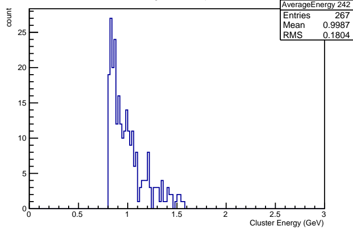
Cluster Energies in Crystal nr 242
