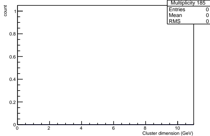
Cluster Dimensions in crystal nr 185
