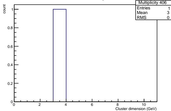
Cluster Dimensions in crystal nr 406
