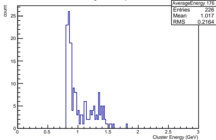
Cluster Energies in Crystal nr 176
