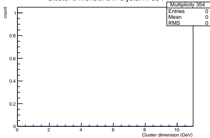
Cluster Dimensions in crystal nr 354
