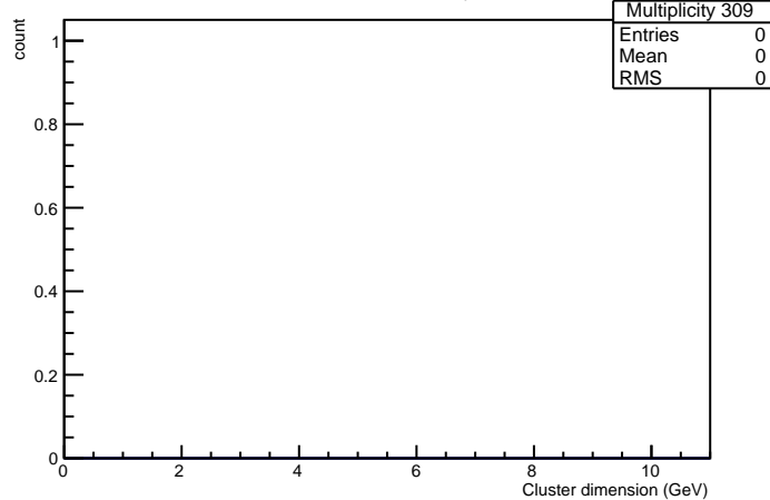
Cluster Dimensions in crystal nr 309
