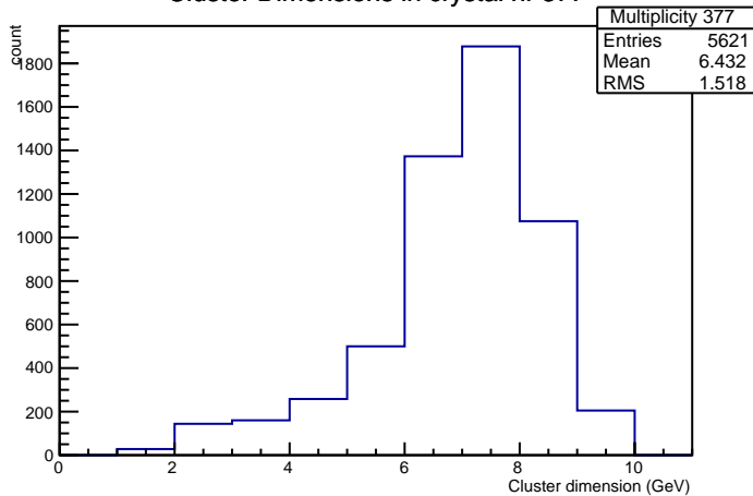
Cluster Dimensions in crystal nr 377
