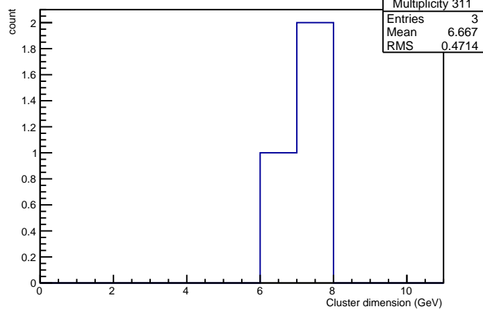
Cluster Dimensions in crystal nr 311
