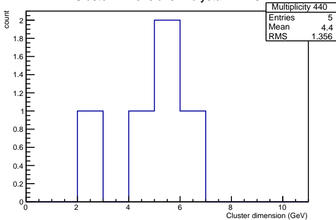
Cluster Dimensions in crystal nr 440
