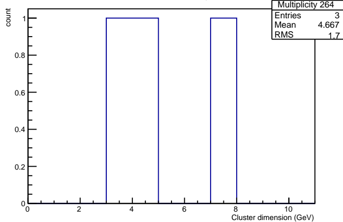
Cluster Dimensions in crystal nr 264
