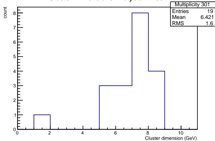
Cluster Dimensions in crystal nr 301
