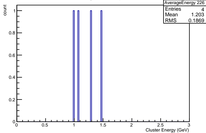
Cluster Energies in Crystal nr 226
