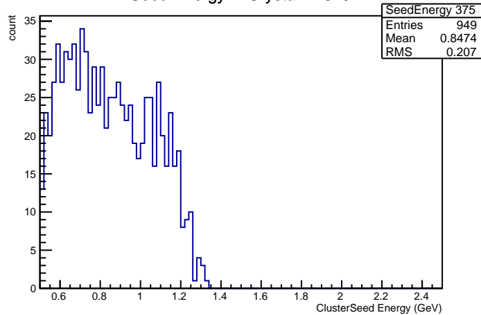
Seed Energy in Crystal nr 375
