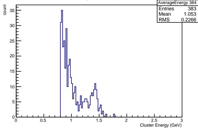
Cluster Energies in Crystal nr 384
