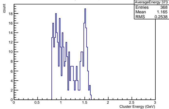
Cluster Energies in Crystal nr 373
