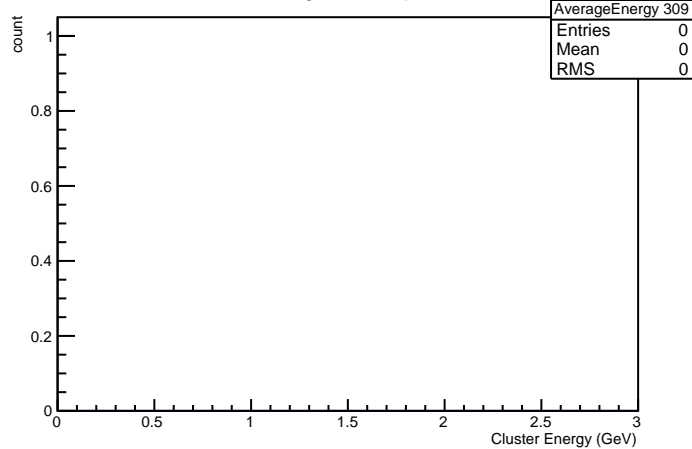
Cluster Energies in Crystal nr 309
