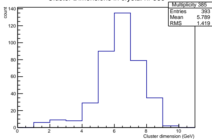
Cluster Dimensions in crystal nr 385
