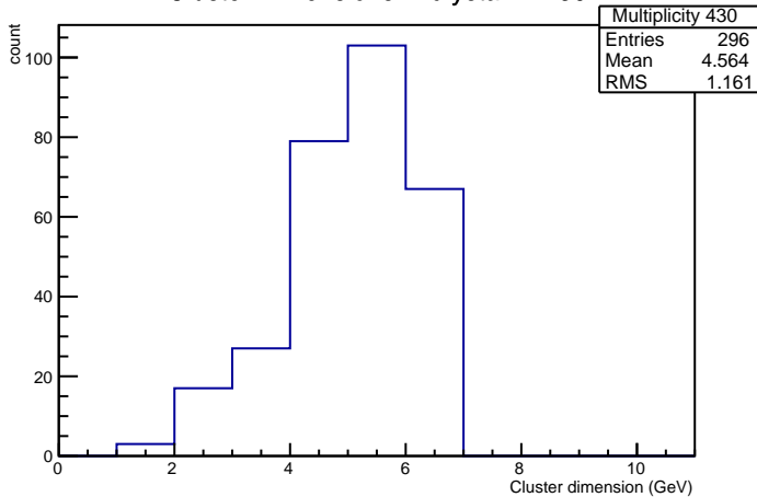
Cluster Dimensions in crystal nr 430
