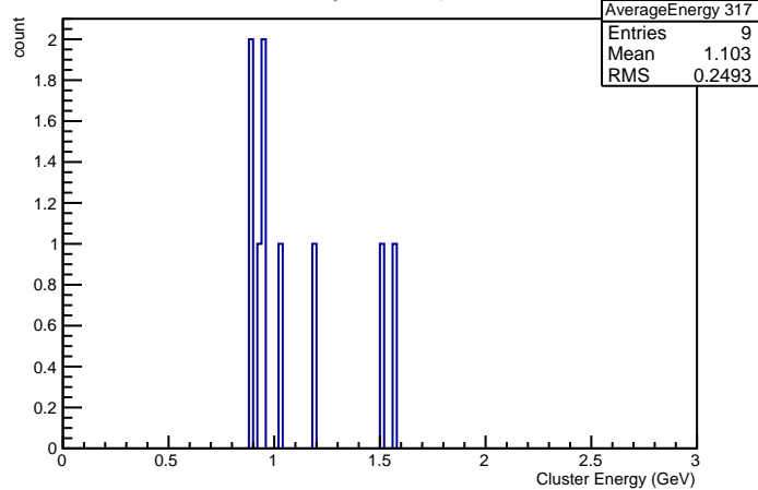
Cluster Energies in Crystal nr 317
