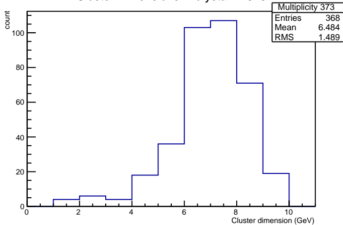
Cluster Dimensions in crystal nr 373
