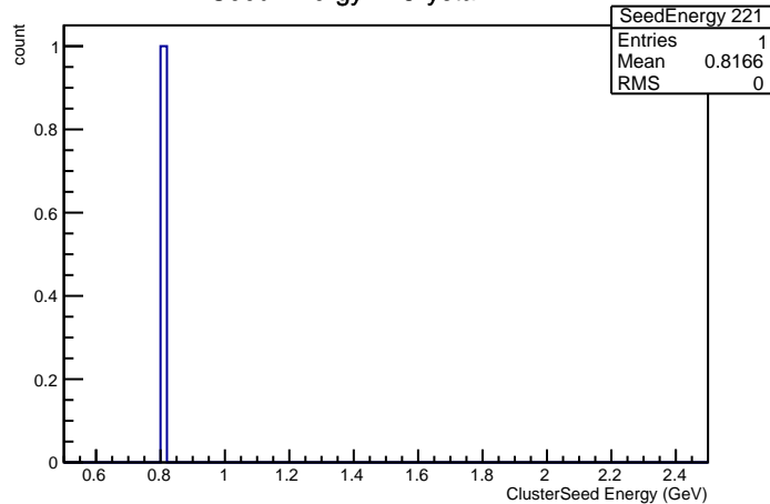
Seed Energy in Crystal nr 221
