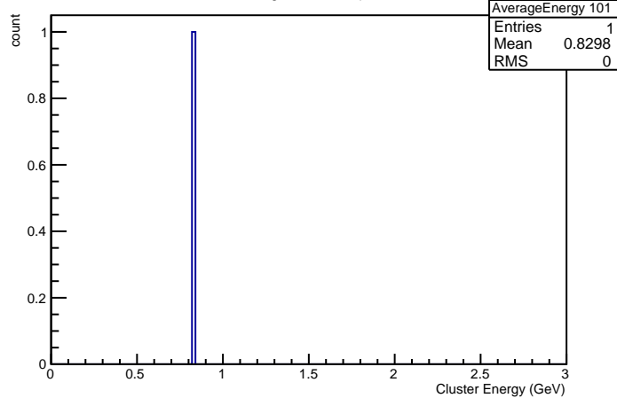
Cluster Energies in Crystal nr 101
