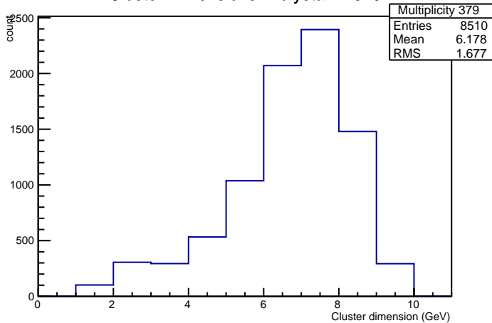
Cluster Dimensions in crystal nr 379
