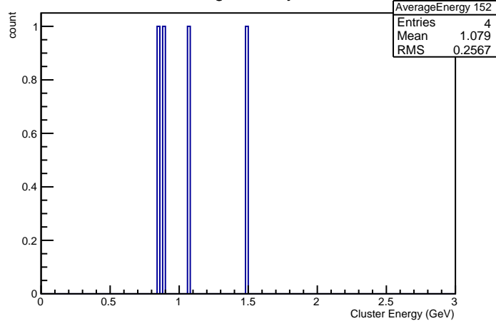
Cluster Energies in Crystal nr 152
