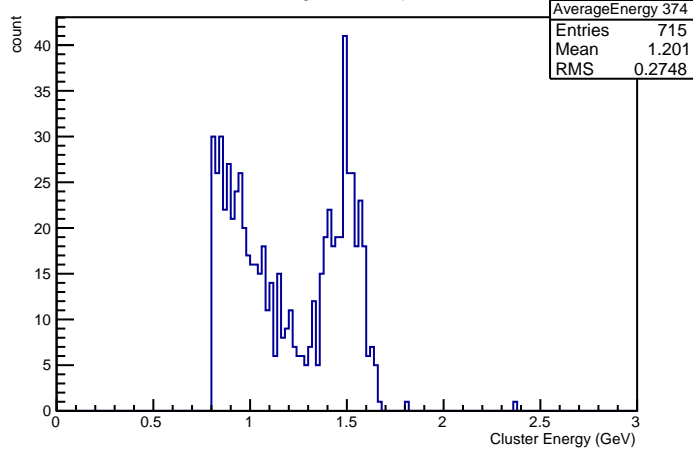
Cluster Energies in Crystal nr 374
