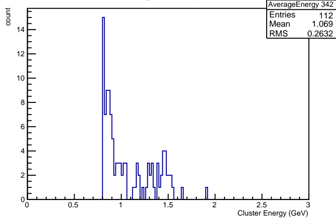
Cluster Energies in Crystal nr 342
