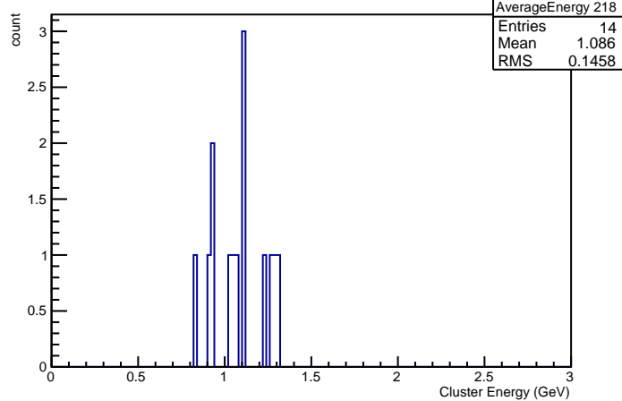
Cluster Energies in Crystal nr 218
