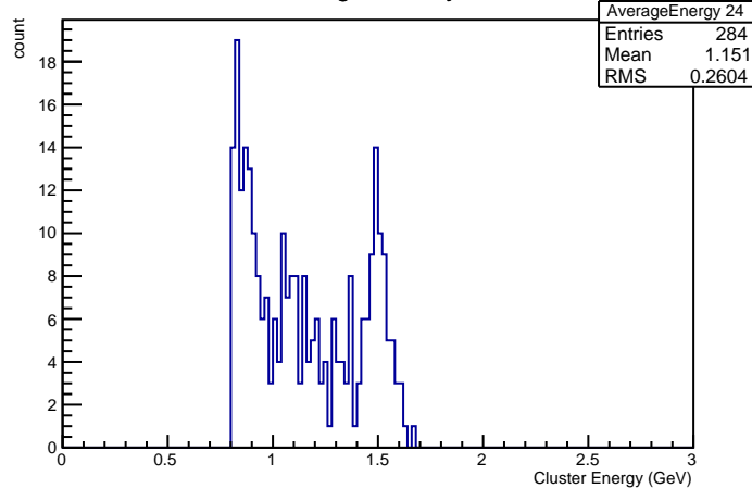
Cluster Energies in Crystal nr 24
