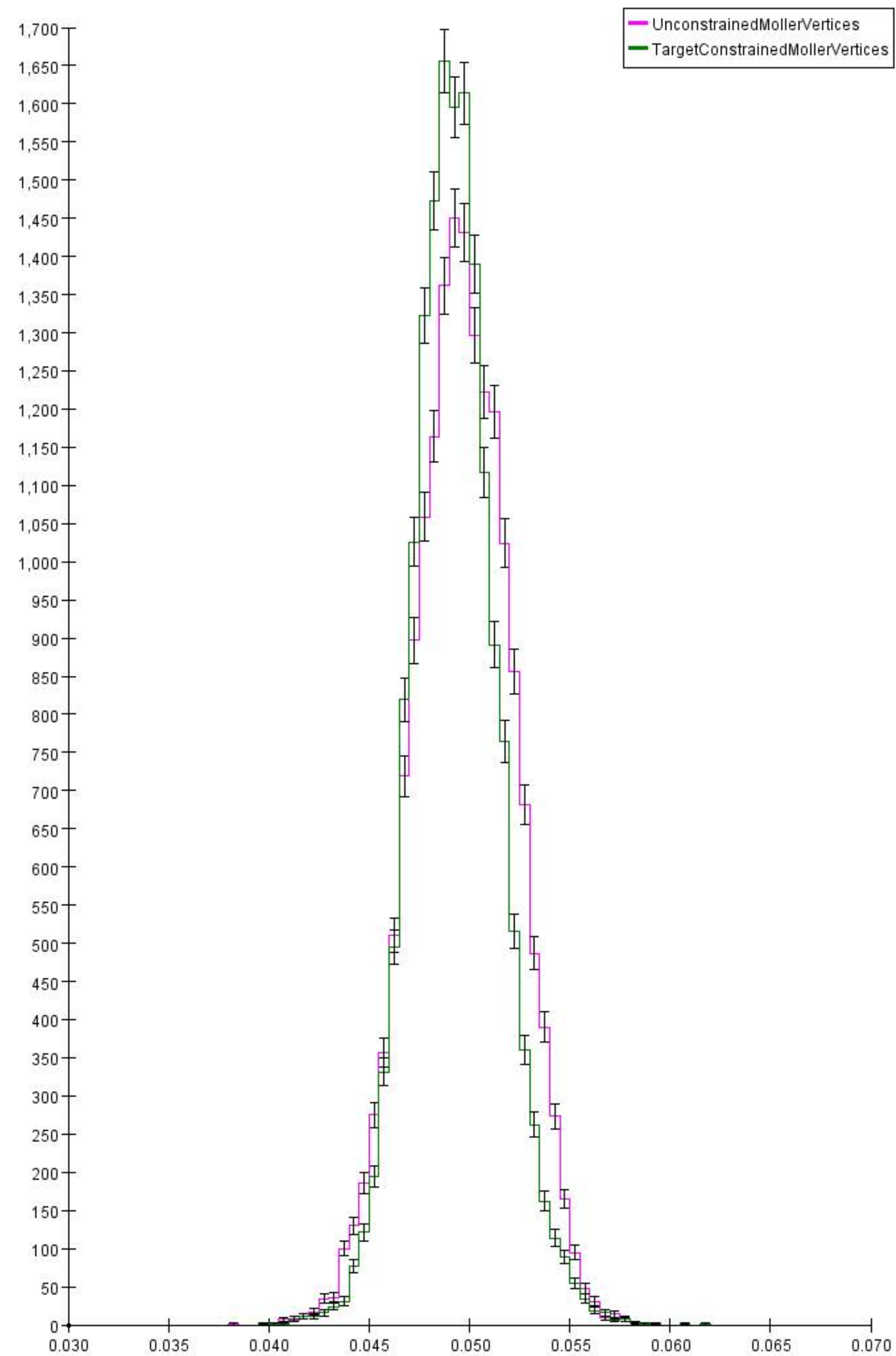
2016Mollerv31.aida - Moller Invariant Mass
