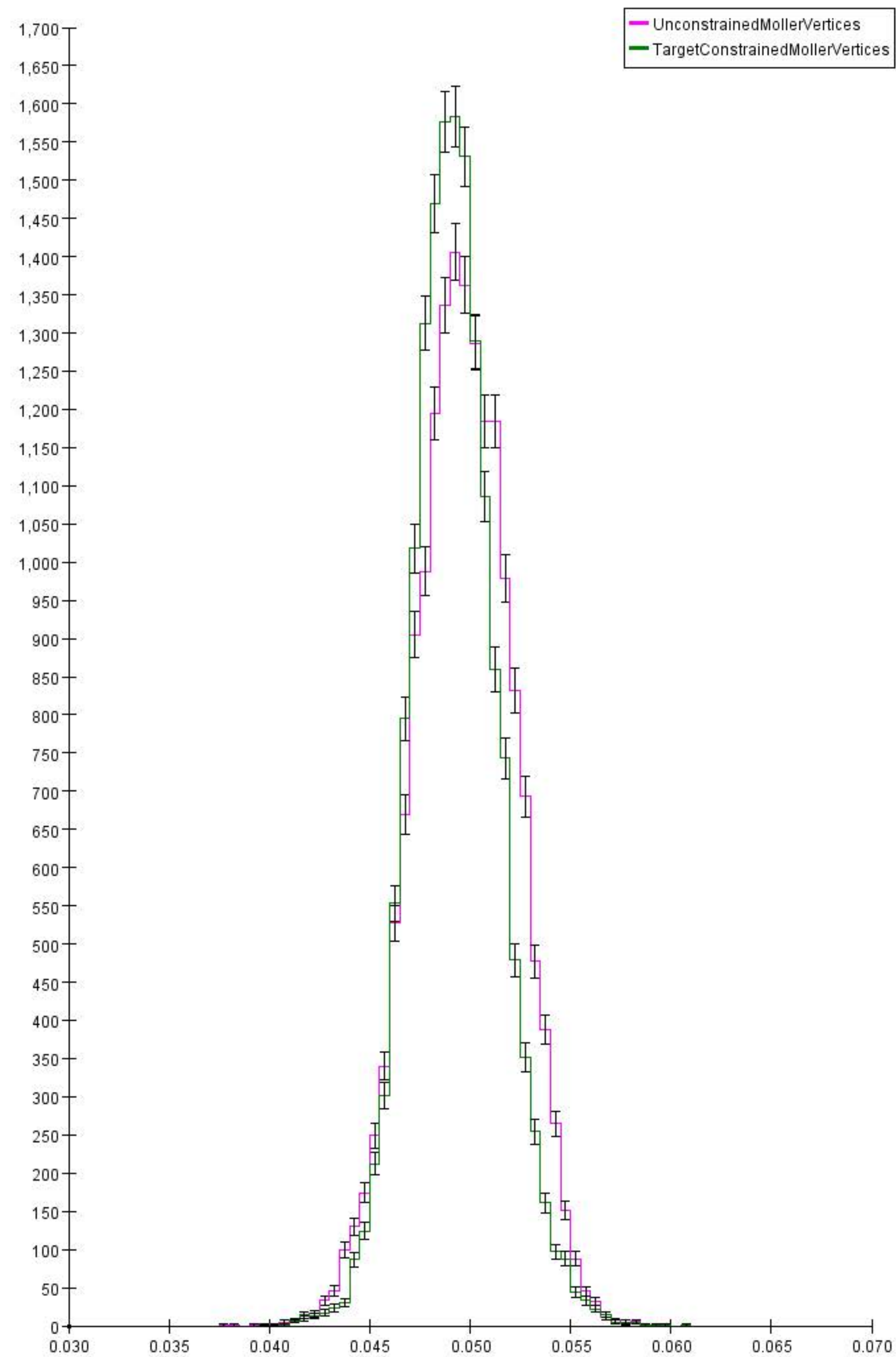
2016Mollerv20.aida - Moller Invariant Mass
